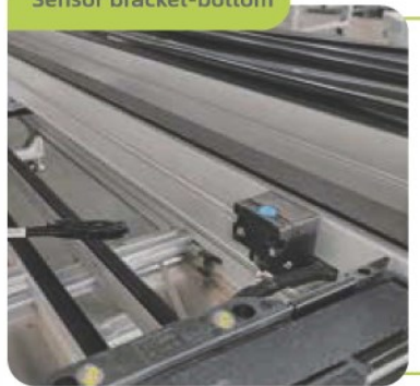
Sensor bracket-bottom
